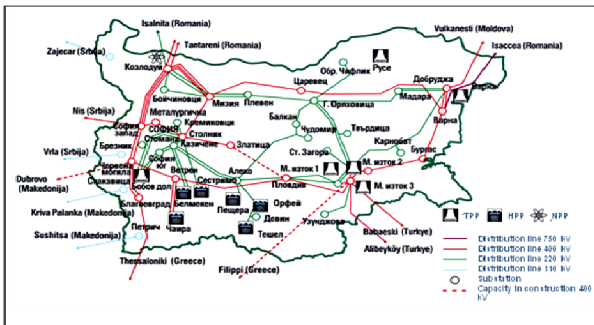
Мрежа високо напрежение в България
